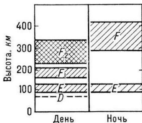
Рисунок 1.3 – Схема вертикального строения ионосферы.
