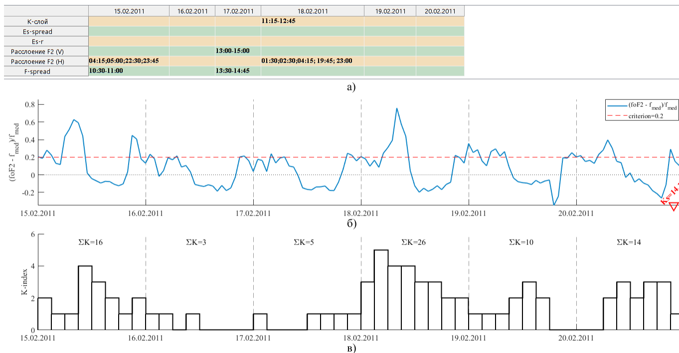
Рисунок Б.4 – Ионосферные и геомагнитный параметры за временной период 15.02.2011–20.02.2011 гг.: а) К-слой, Es-spread, Es типа r, расслоение F2 (режим V), расслоение F2 (режим H), F-spread; б) часовые значения параметра \Delta foF2/f_{med} (на временной оси отмечено землетрясение с K_S = 14.1 ); в) трёхчасовые значения индекса геомагнитной активности K .
