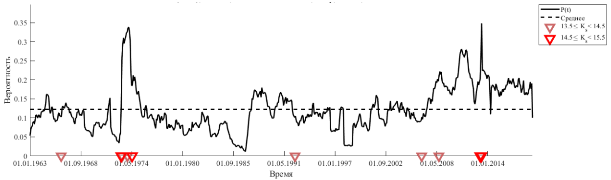
Рисунок А.1 – Временной ряд значений вероятности P_k(S_1) .
