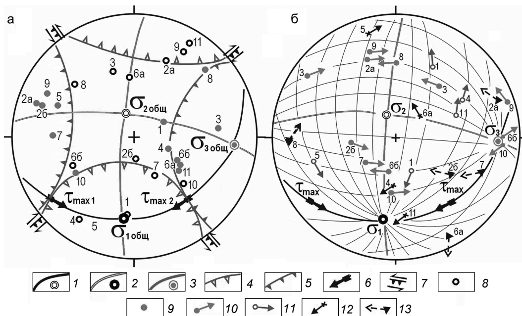
Рис. 3. Стереогаммы неотектонических напряжений Южного Сахалина.
